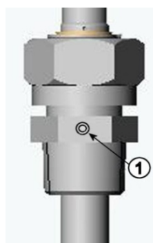
图 28 DMT348 探头中的放气螺钉
